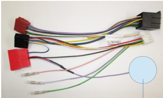
Označení kabelového svazku: C-3474261
