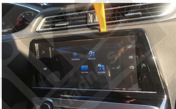
2. Demontujte rámeček obrazovky
